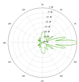
H-Plane, 3550 MHz
